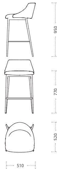
Sgabello High stool
